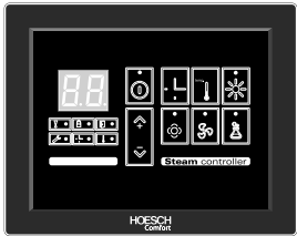
额外非防水的控制面板，用于安装在蒸气房/蒸汽浴室外。商品编号6832
