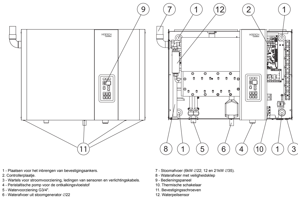
Fig.1 Bouw van de stoomgenerator
