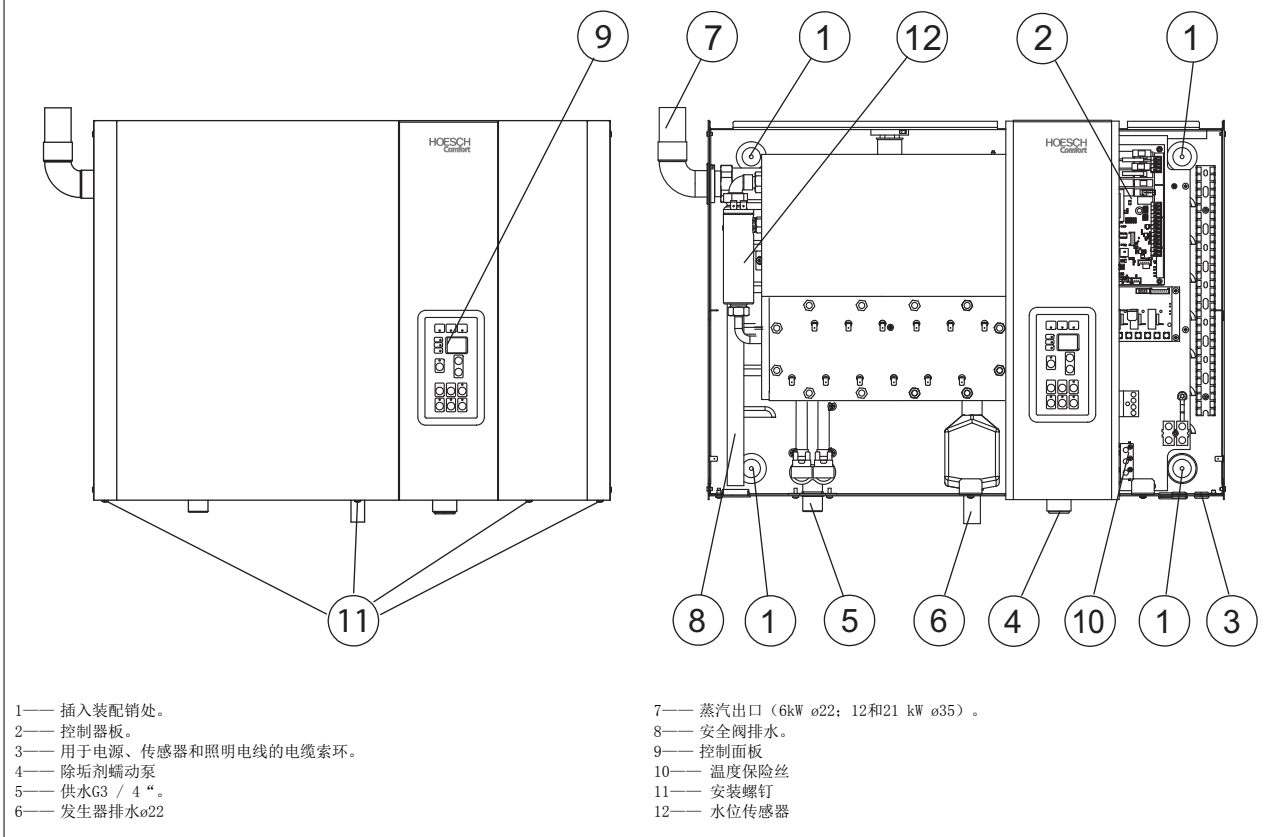
图1 蒸汽发生器的结构
