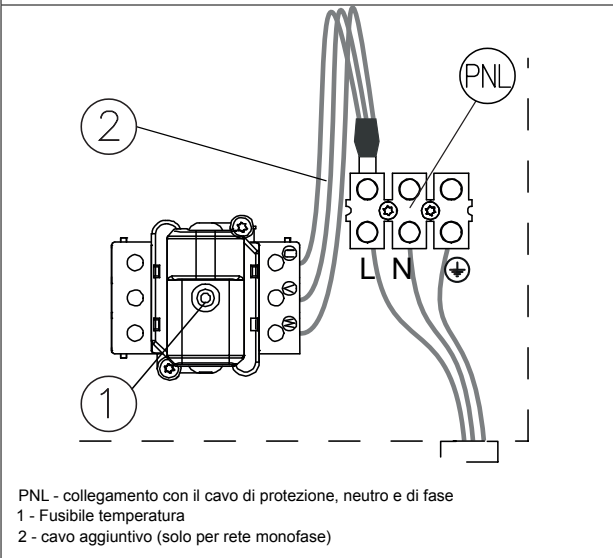
Fig.4.2 Collegamento all'impianto monofase (Hoesch 6)
