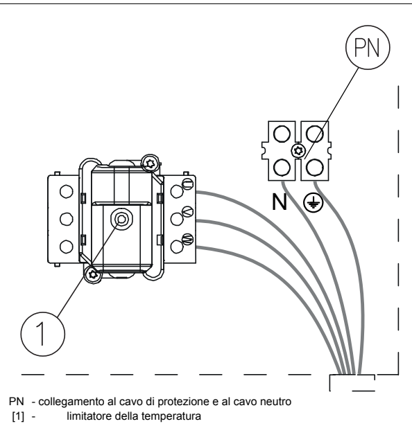
Fig. 4.3 Collegamento all'impianto trifase (Hoesch 6, Hoesch 12, Hoesch 21)
