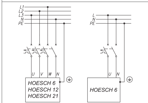
Abb. 4.1 Anschlusschema
