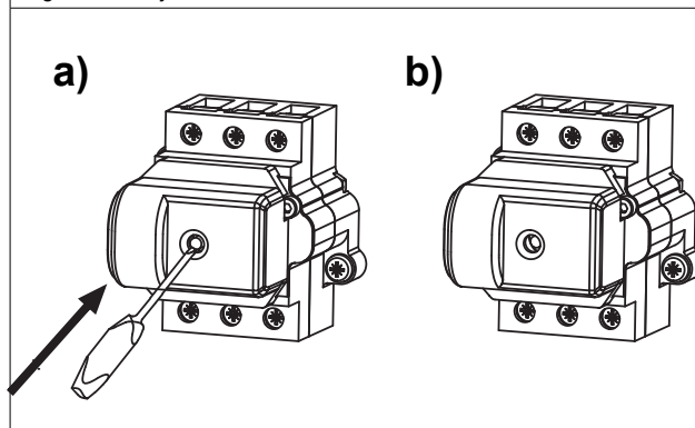
Fig.4.4 Disjoncteur WT3a
