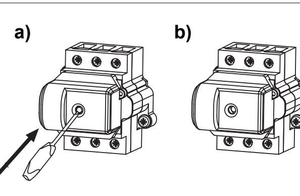
Fig. 4.4 Interruttore WT3a
