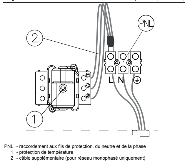
Figure 4.2 Raccordement à une installation monophasée (Hoesch 6)
