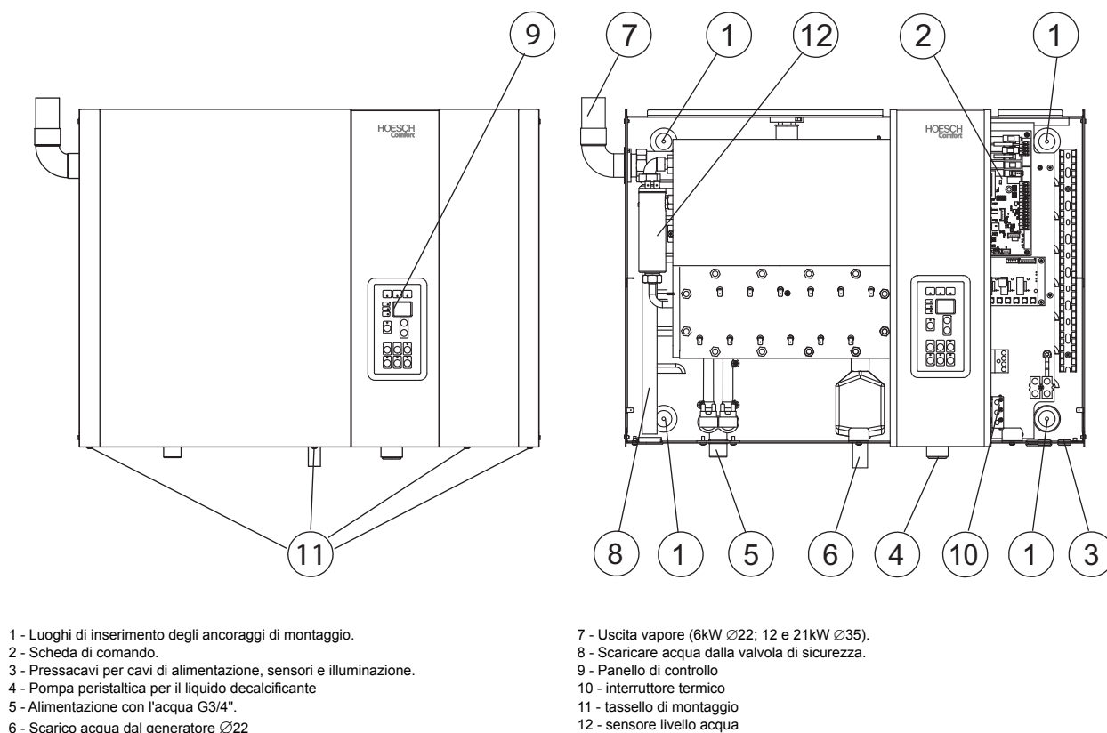
Fig.1 Struttura del generatore di vapore
