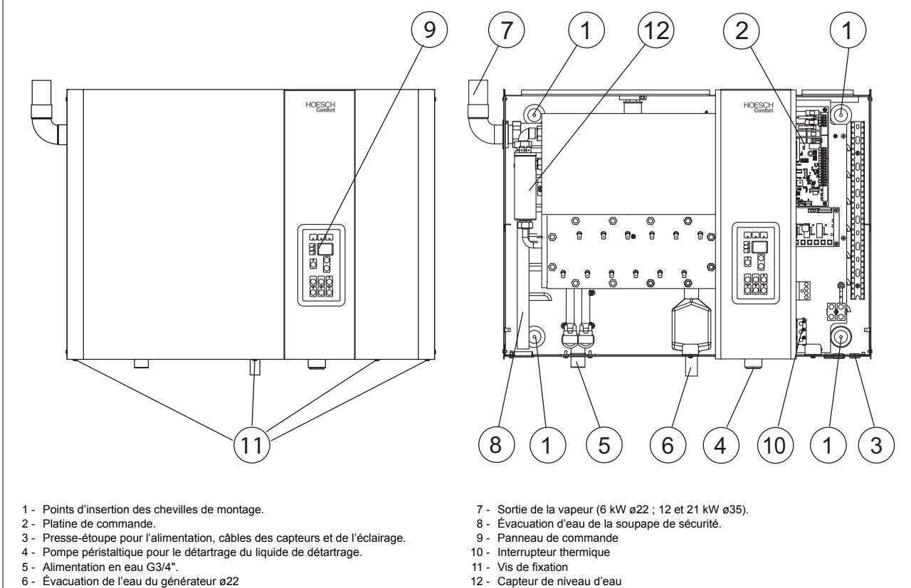
Fig.1 Conception du générateur de vapeur
