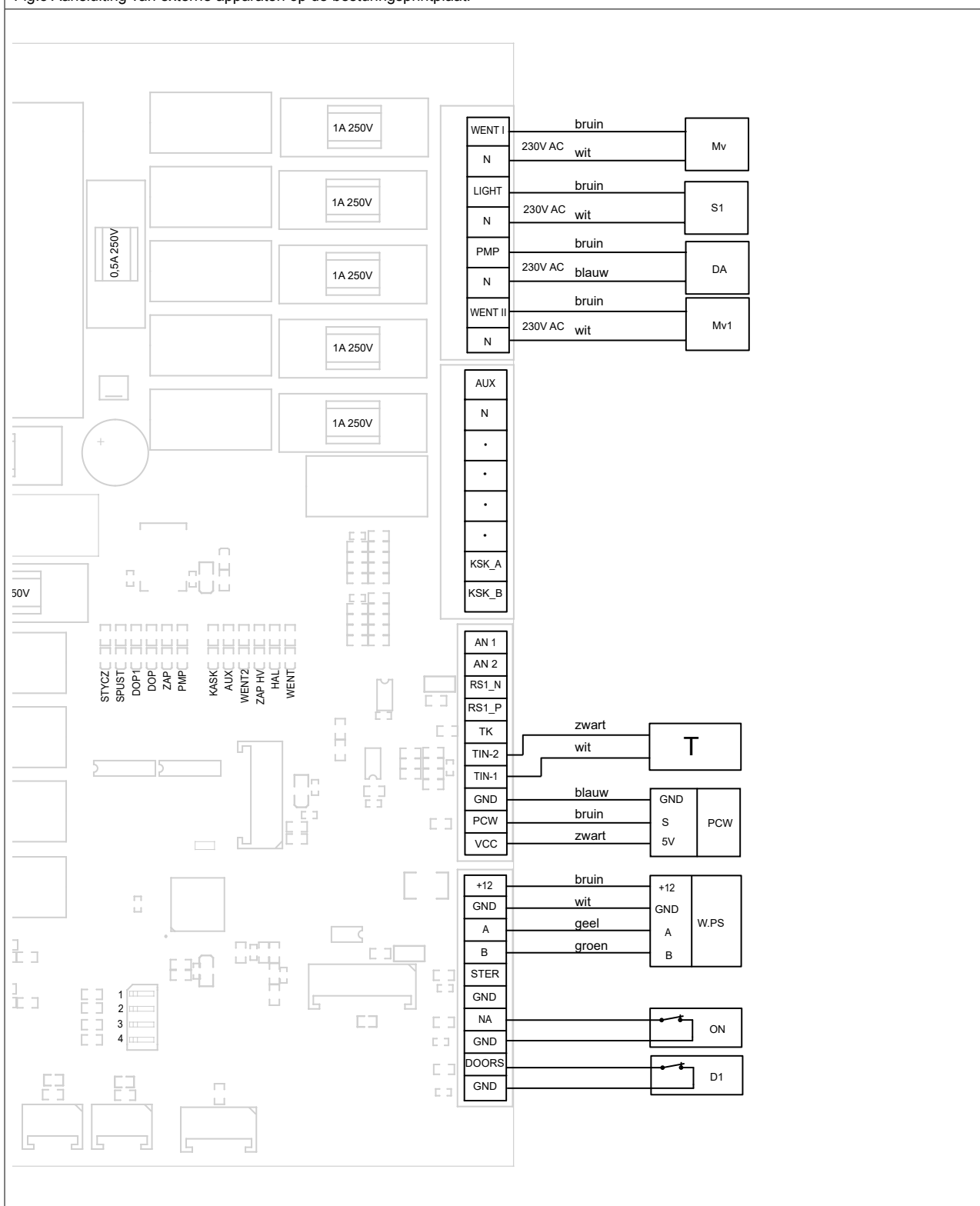
Fig.5 Aansluiting van externe apparaten op de besturingsprintplaat.
