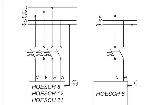
Рис.4.1 Схема подключения
