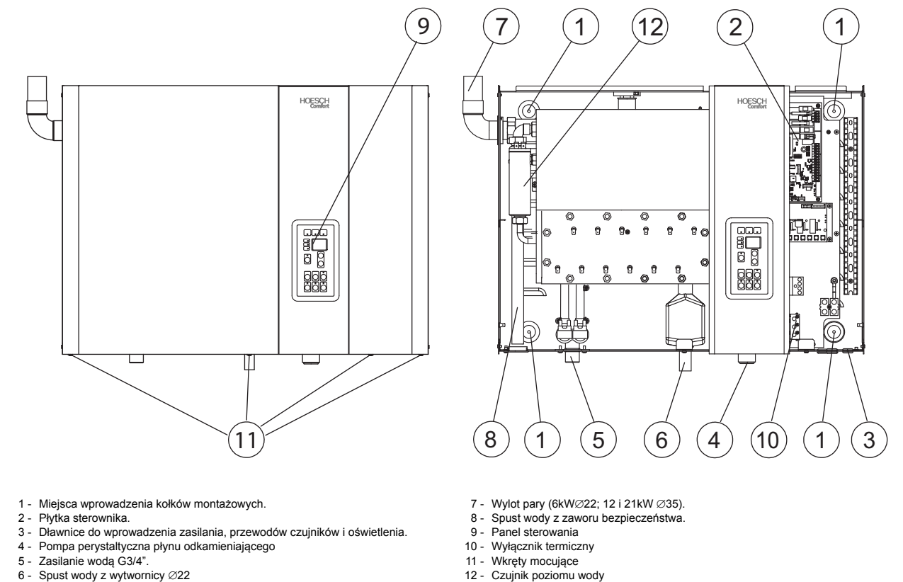
Rys.1 Konstrukcja wytwornicy pary
