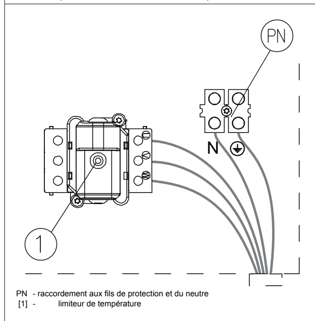
Figure 4.3 Raccordement à une installation triphasé (Hoesch 6, Hoesch 12, Hoesch 21)
