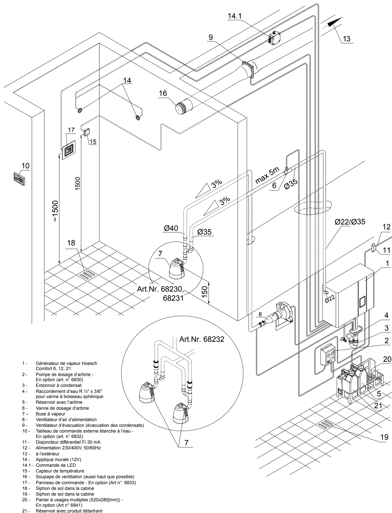
Illustration du schéma du système de bain de vapeur variante 2 - générateur sous le niveau du bain de vapeur
