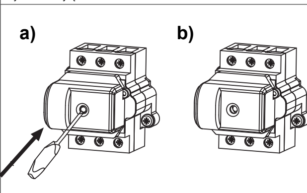
Rys.4.4 Wyłącznik WT3a
