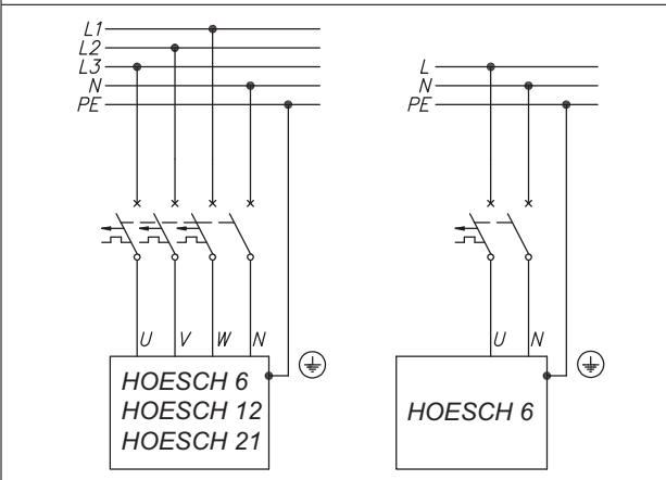
Fig.4.1 Schema di collegamento
