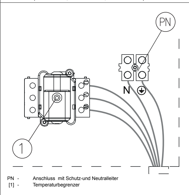
Abb. 4.3 Anschluss dreiphasig (HOESCH 6, HOESCH 12, HOESCH 21)
