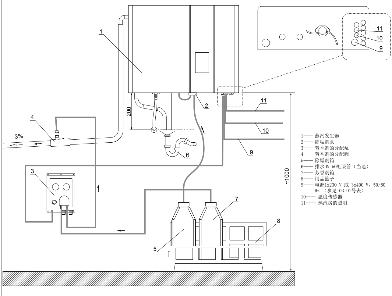
图2 蒸汽浴中的液压装置和温度传感器
