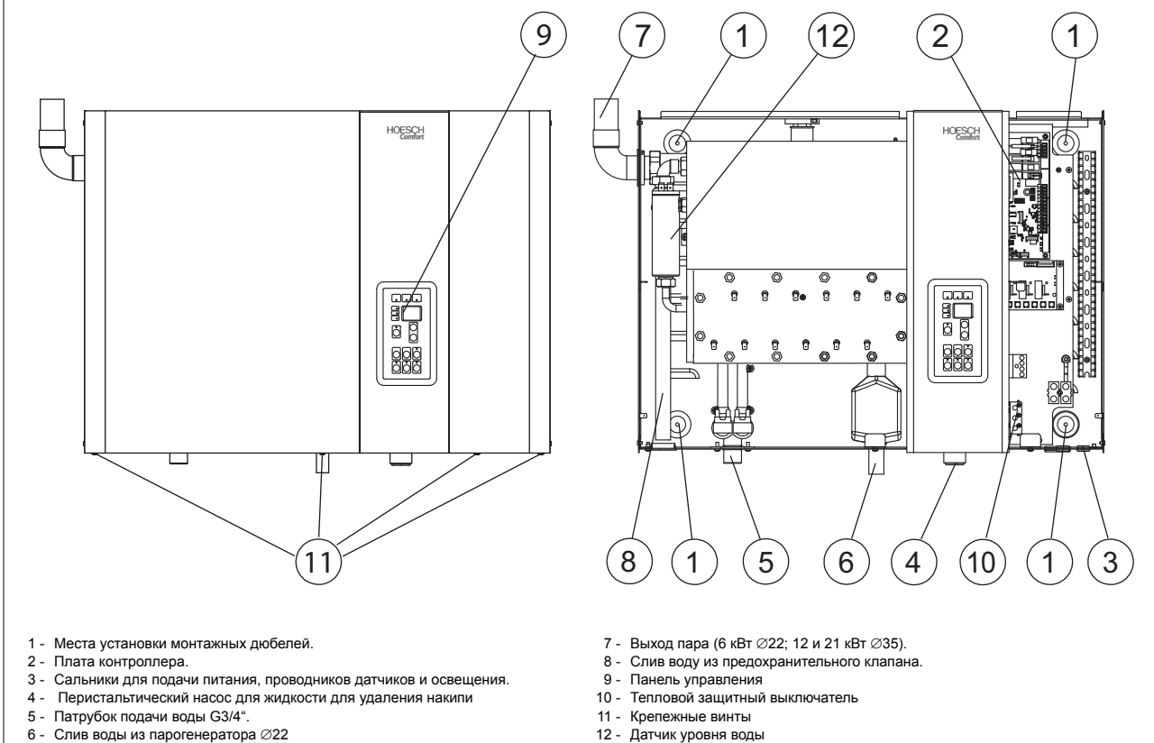
Рис.1 Конструкция парогенератора
