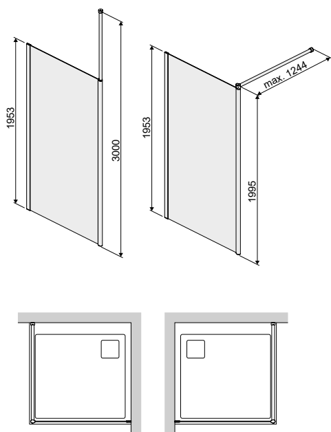
Corner version, side entry / Угловая версия, боковой вход / 转角式侧面入口
