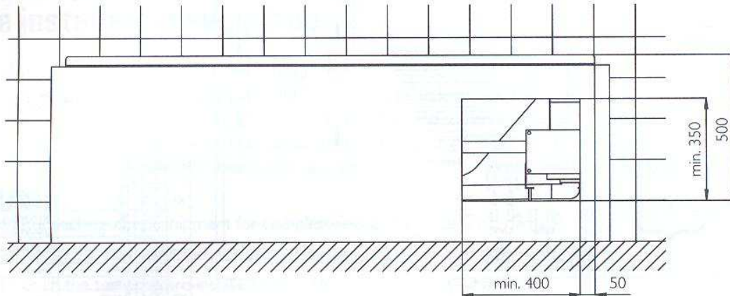
Erforderliche Revisionsöffnung Steuerung/Pumpe
