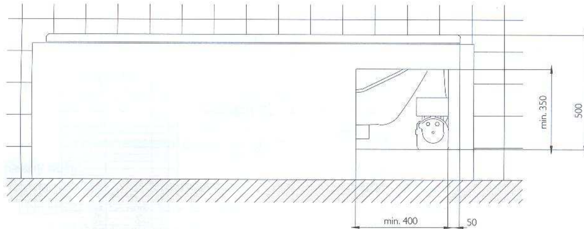
Erforderliche Revisionsöffnung Steuerung/Gebläse
